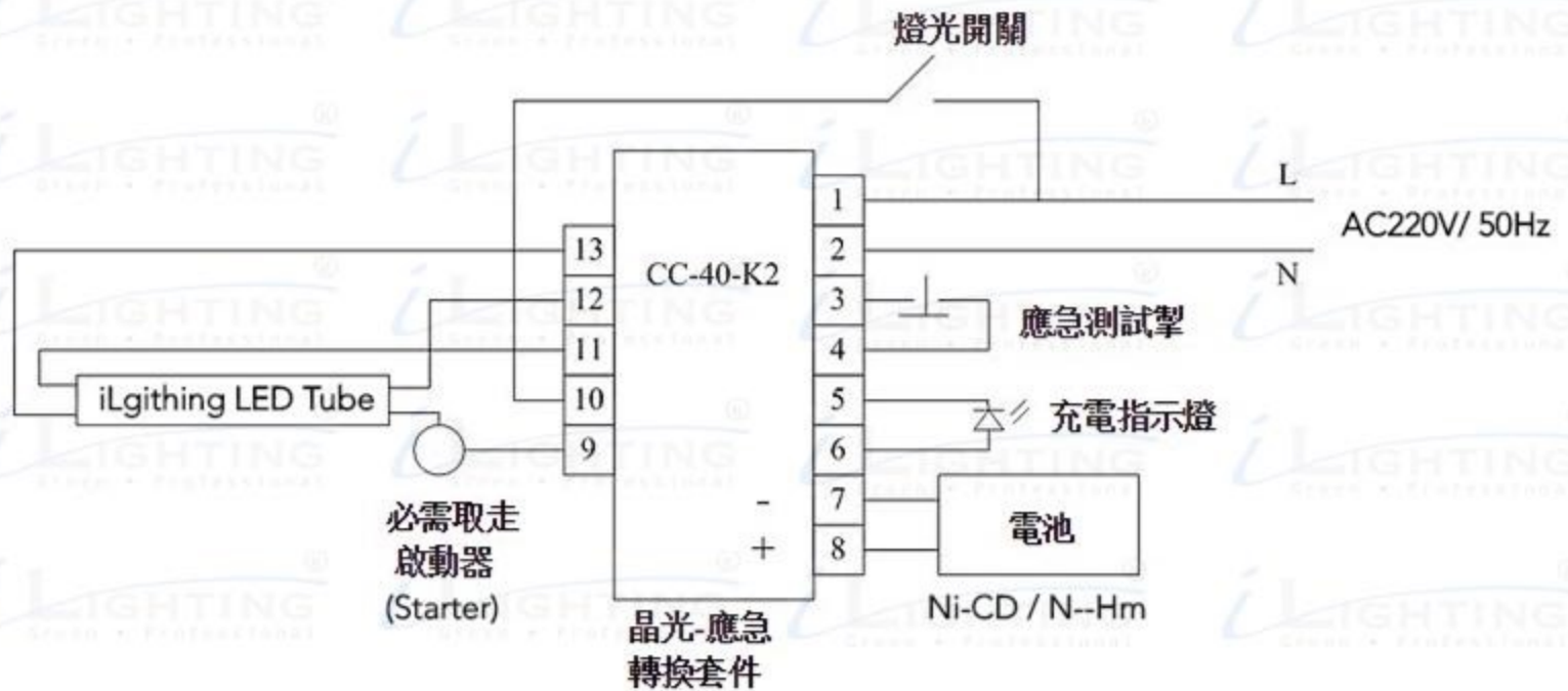
舊T8支架應急支架改造接線圖 CC 40-k2 - ( EM Ballast )
