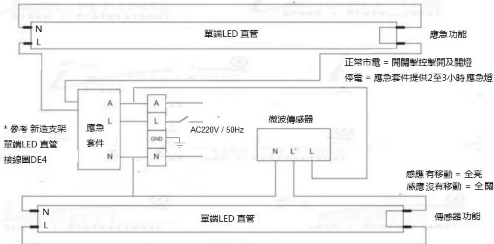
新T8雙T8支架 帶微波傳感器和應急套件接線圖
