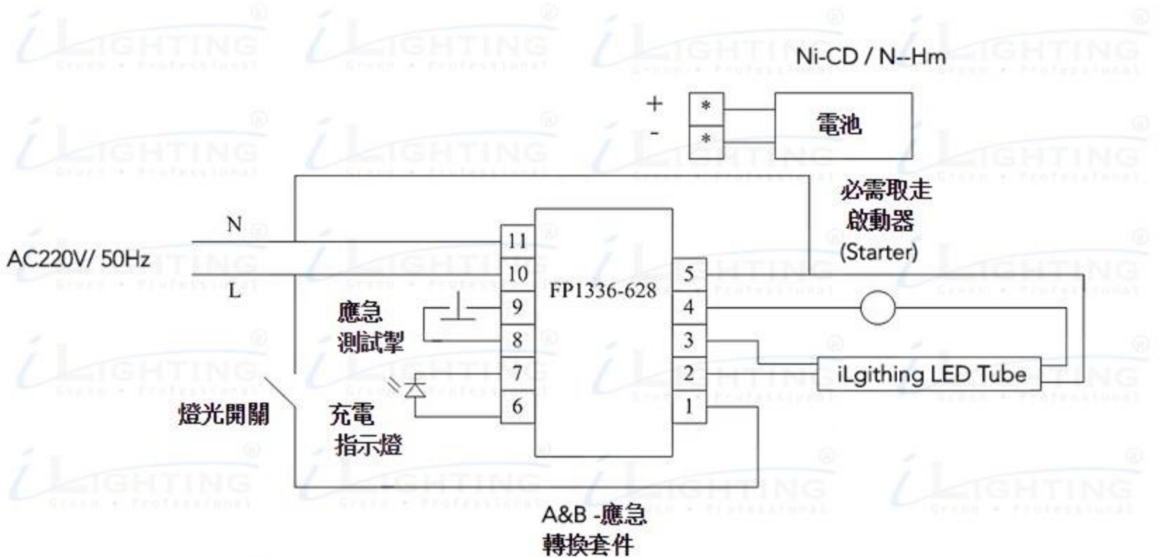
舊T8支應急支架改造接線圖接線圖 FP-1336-628 - (EM Ballast)
