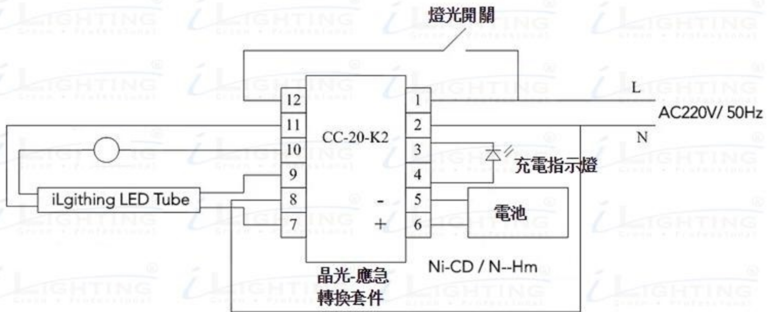
舊T8支架應急支架改造接線圖 CC 20-k2 - ( EM Ballast )
